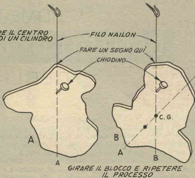
COME SI TROVA IL CENTRO DI GRAVITA' DI UN OGGETTO CON CONTORNI IRREGOLARI MA DI SPESSORE COSTANTE
