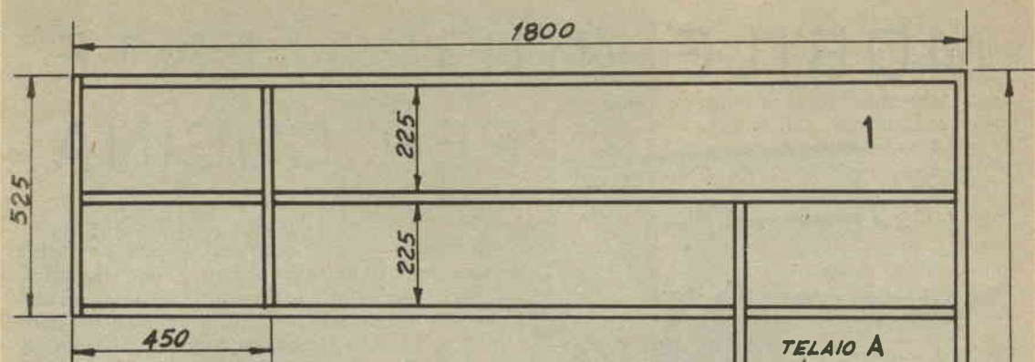
Fig. 1 - Veduta generale delle dimensioni e dei rapporti delle strutture
